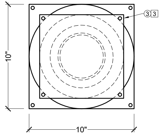
TOP VIEW SCALE: \frac{3}{16}'' = 1''
