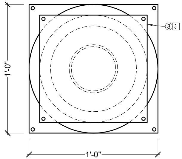
TOP VIEW SCALE: \frac{3}{16} " = 1"
