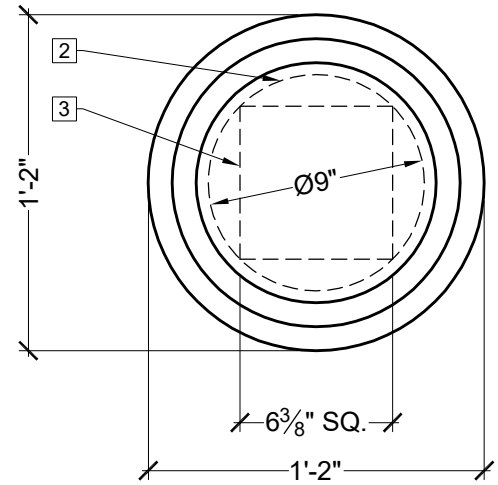
TOP VIEW SCALE: 3/8" = 1"
