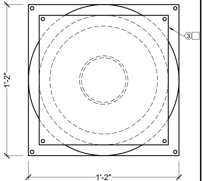
TOP VIEW SCALE: \frac{3}{16}'' = 1''
