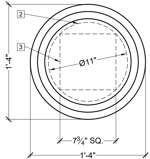
TOP VIEW SCALE: 1/8" = 1"
