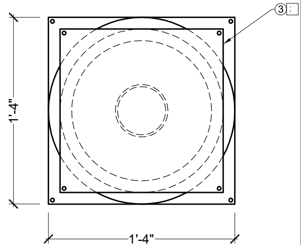
TOP VIEW SCALE: 1/8" = 1"
