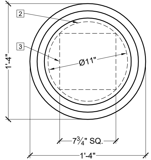
TOP VIEW SCALE: \frac{5}{8}'' = 1''
