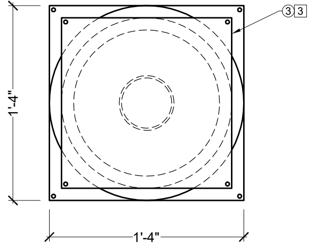
TOP VIEW SCALE: \frac{5}{8}'' = 1''
