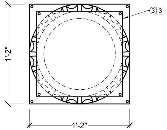
TOP VIEW SCALE: \frac{1}{8}'' = 1''
