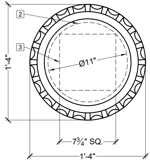
TOP VIEW SCALE: 3/8" = 1"
