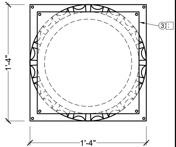
TOP VIEW SCALE: 5/8" = 1"
