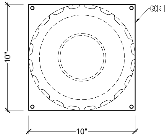
TOP VIEW SCALE: \frac{5}{16}'' = 1''
