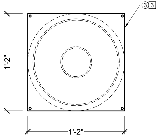
TOP VIEW SCALE: 5/8" = 1"
