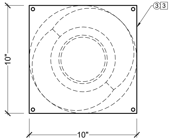
TOP VIEW SCALE: \frac{3}{16}'' = 1''
